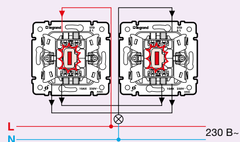
Переключатель на 2 направления с подсветкой (управление с 2-х мест) Кат. № 7 744 26 - 7 743 26 - 7 701 26
