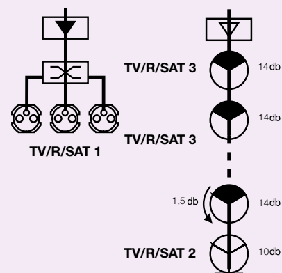
TV/R/SAT 1/2/3
