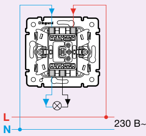
Двухполюсный выключатель Кат. № 7 744 02 - 7 743 02 - 7 701 02
