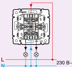
Выключатель двухклавишный с индикацией Кат. № 7 744 45 - 7 743 45 - 7 701 45 6 942 78 - 6 956 06
