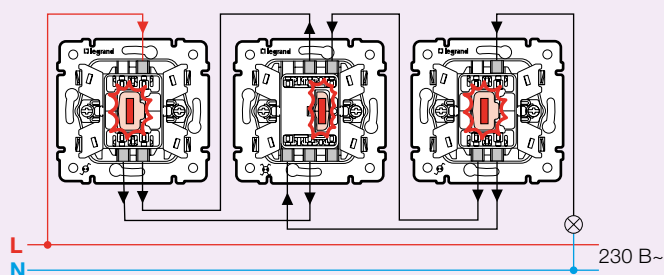
Переключатели на 2 направления и промежуточный переключатель с подсветкой (управление с 3-х мест) 7 743 26 + 7 743 48 + 7 743 26 (или 7 744 26 + 7 744 48 + 7 744 26)
