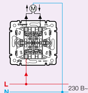
Переключатель без фиксации с электрической блокировкой для управления приводами рольставней Кат. № 7 744 14 - 7 743 14 - 7 701 14
