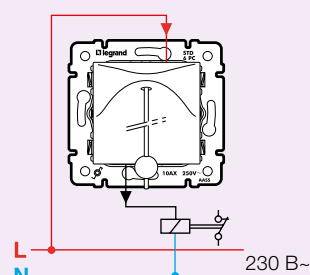
Переключатель без фиксации перекидной со шнуром Кат. № 7 744 19 - 7 743 19 - 7 701 19
