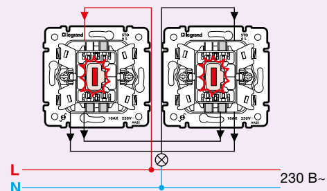
Переключатель на 2 направления с подсветкой (управление с 2-х мест) Кат. № 7 744 26 - 7 743 26 - 7 701 26
