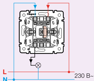
Переключатель на 2 направления с индикацией Кат. № 7 744 25 - 7 743 25 - 7 701 25
