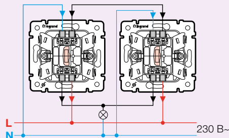
Переключатель на 2 направления с индикацией (управление с 2-х мест) Кат. № 7 744 25 - 7 743 25 - 7 701 25
