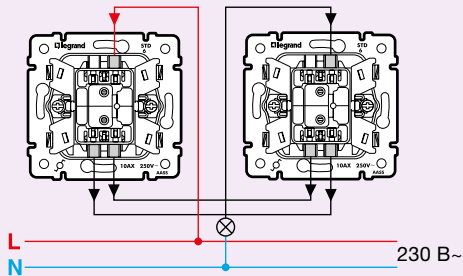
Переключатель на два направления (управление с 2-х мест) Кат. № 7 744 06 - 7 743 06 - 7 701 06 6 942 62 - 6 956 02 - 6 943 38
