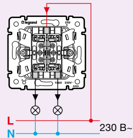
Выключатель двухклавишный Кат. № 7 744 05 - 7 743 05 - 7 701 05 6 942 65 - 6 956 05 - 6 943 37
