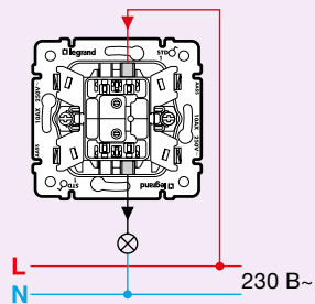
Выключатель Кат. № 7 744 01 - 7 743 01 - 7 701 01 6 942 60 - 6 956 00 - 6 943 36
