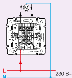
Переключатель с механической блокировкой для управления приводами рольставней Кат. № 7 744 04 - 7 743 04 - 7 701 04
