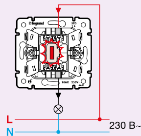
Выключатель с подсветкой Кат. № 7 744 10 - 7 743 10 - 7 701 10 6 942 61 - 6 956 01 - 6 943 40
