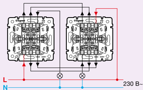
Переключатель двухклавишный два направления (управление двумя нагрузками с 2-х мест) Кат. № 7 744 08 - 7 743 08 - 7 701 08 6 942 66 - 6 956 04 - 6 943 39
