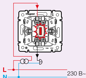
Выключатель без фиксации с подсветкой (с символом звонка) Кат. № 7 744 15 - 7 743 15 - 7 701 15
