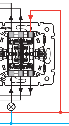
STD 6/2 - 6/2 IP44
