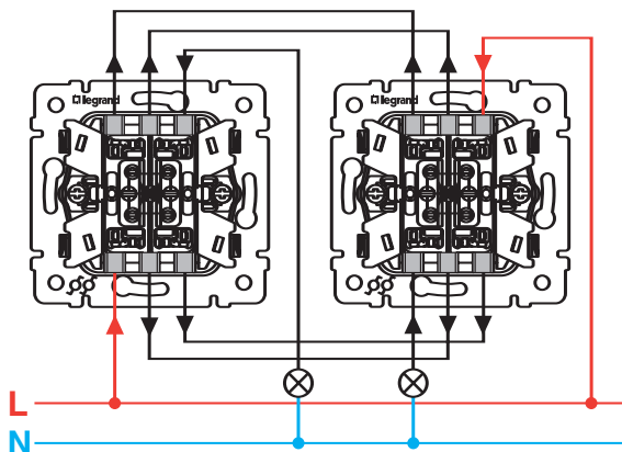
STD 6/2 - 6/2 IP44
